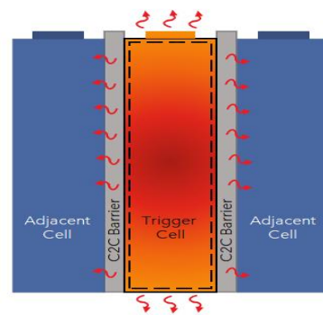
그림 46. 열폭주방지패드 - 1,000°C 이상에서도 효과적 열 저항
