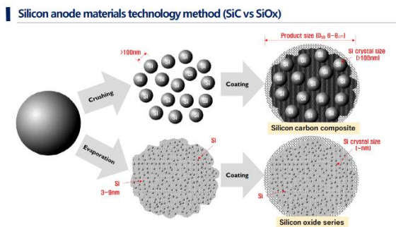
그림 43. Si-Ox vs SiC 입자 크기 비교
