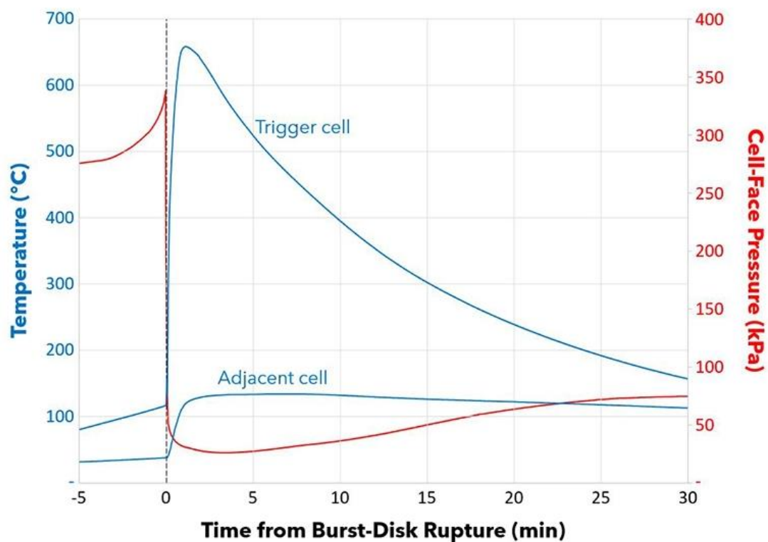
그림 47. Aspen Aerogel PYROTHIN 열폭주방지패드 적용 사례 - 화재 시 Trigger Cell 과 Adjacent Cell 의 온도변화 추이
